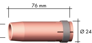
ABIMIG® GRIP W 555 (VE=10)
